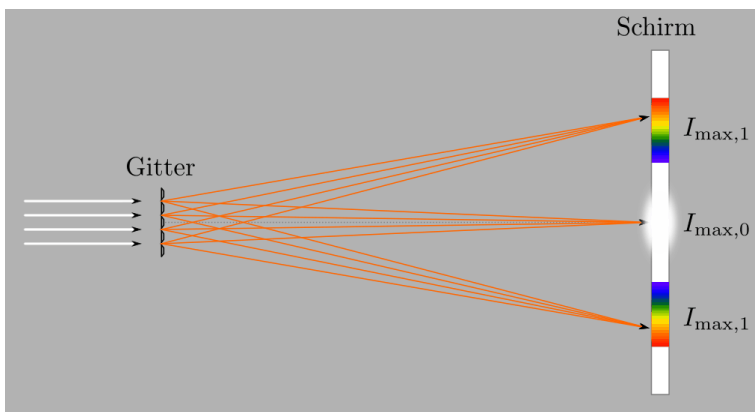
Abb. 3.38 Interferenzmaxima am optischen Gitter.
