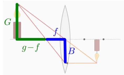
Abb. 3.25 Herleitung der Linsengleichung (Strahlensatz).
