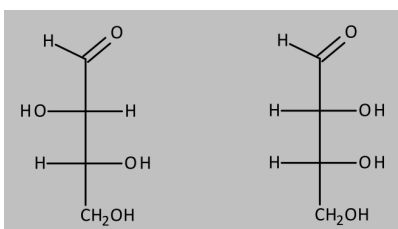
D-Threose D-Erythrose Abb. 9.3. Beispiele für Tetrosen
