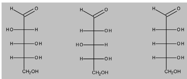
D-Arabinose D-Xylose D-Ribose Abb. 9.2. Beispiele für Monosaccharide mit 5 C-Atomen (Pentosen).
