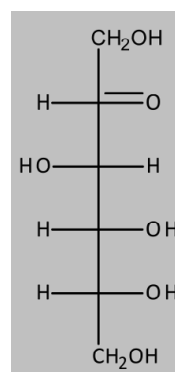
Abb. 9.4. D-Fructose
