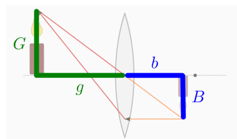
Abb. 3.24 Herleitung der Abbildungsformel (Strahlensatz).
