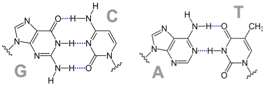
Abb. 9.22: Die Basenpaarung
