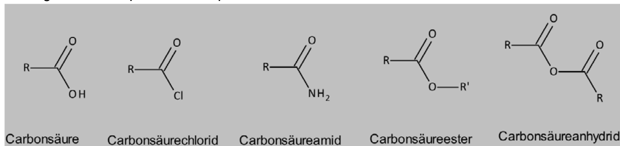
Abb. 7.13: Carbonsäurederivate
