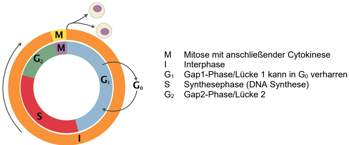
Abb. 2.2: Der Zellzyklus
