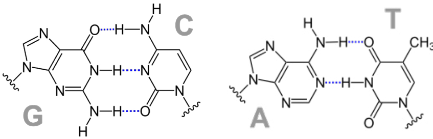
Abb. 9.22: Die Basenpaarung
