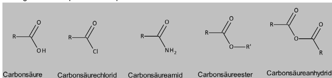
Abb. 7.13: Carbonsäurenderivate
