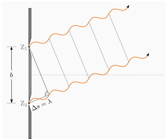
Abb. 3.35a Konstruktive Interferenz am Doppelspalt
