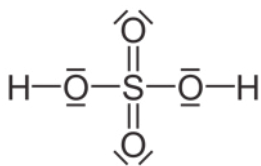
Abb. 3.4: Schwefelsäure (Summenformel: H_2SO_4 ) einschließlich der Außenelektronen
